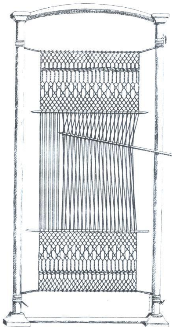
Abb. 247. Gerät zum Flechten in Sprangtechnik.
